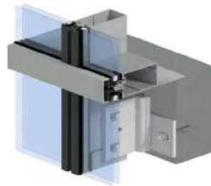
PERFIL HORIZONTAL VISTO Y PERFIL HORIZONTAL OCULTO Y PERFIL VERTICAL OCULTO
