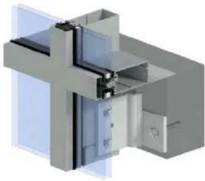
PERFIL HORIZONTAL VISTO Y PERFIL VERTICAL VISTO
