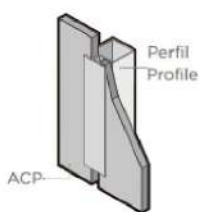
Por inserción
