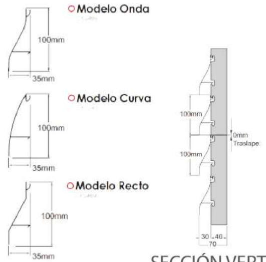
SECCIÓN VERTICAL
