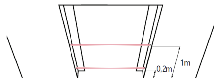
Barrera doble
