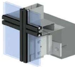
PERFIL HORIZONTAL Y PERFIL VERTICAL OCULTO
