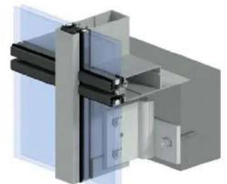
PERFIL HORIZONTAL VISTO Y PERFIL HORIZONTAL OCULTO Y PERFIL VERTICAL OCULTO
